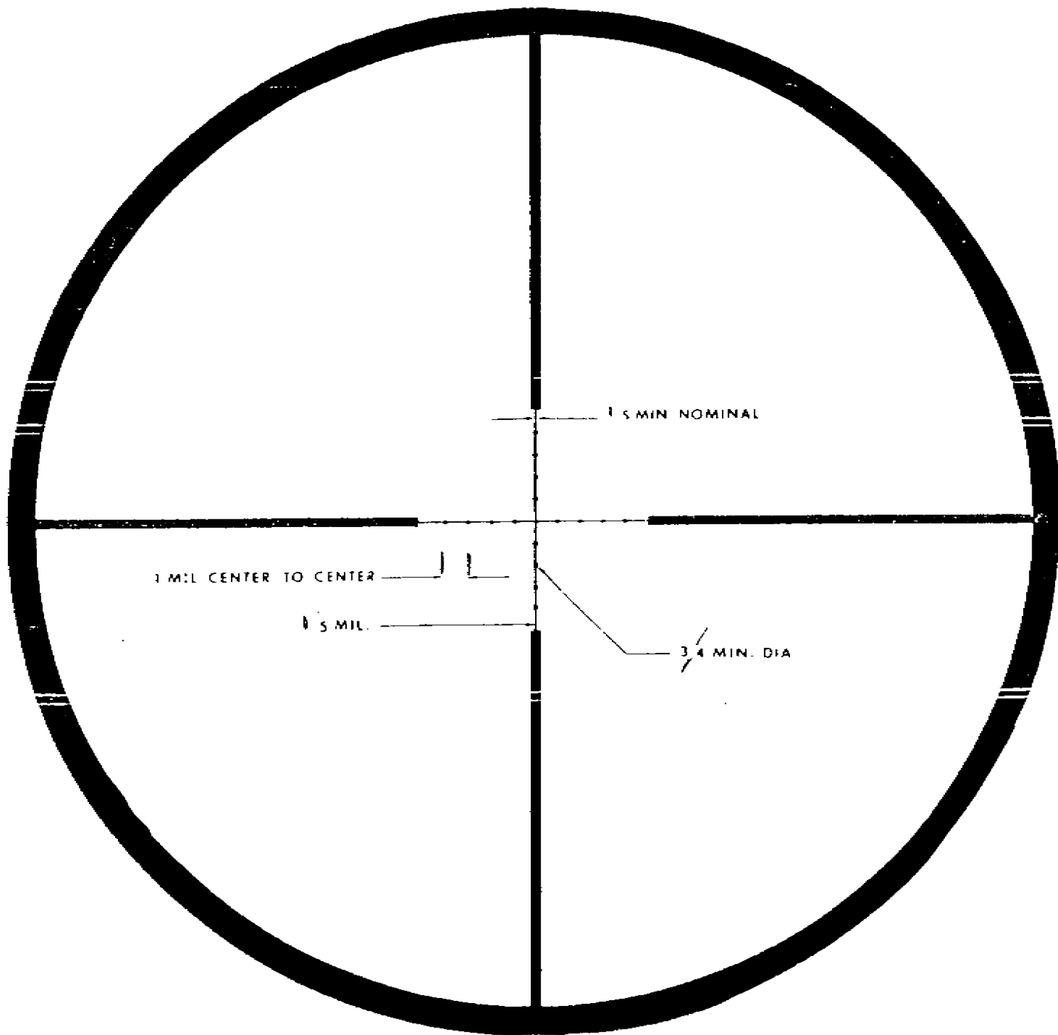
3/4 Min. Mil Dot Reticle Fig. #3
